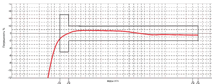
Кривая погрешности
